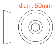
Êmbolo polipropileno
